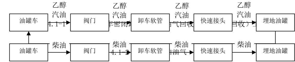
图 2.4.1-3 乙醇汽油加油及油气回收流程图
