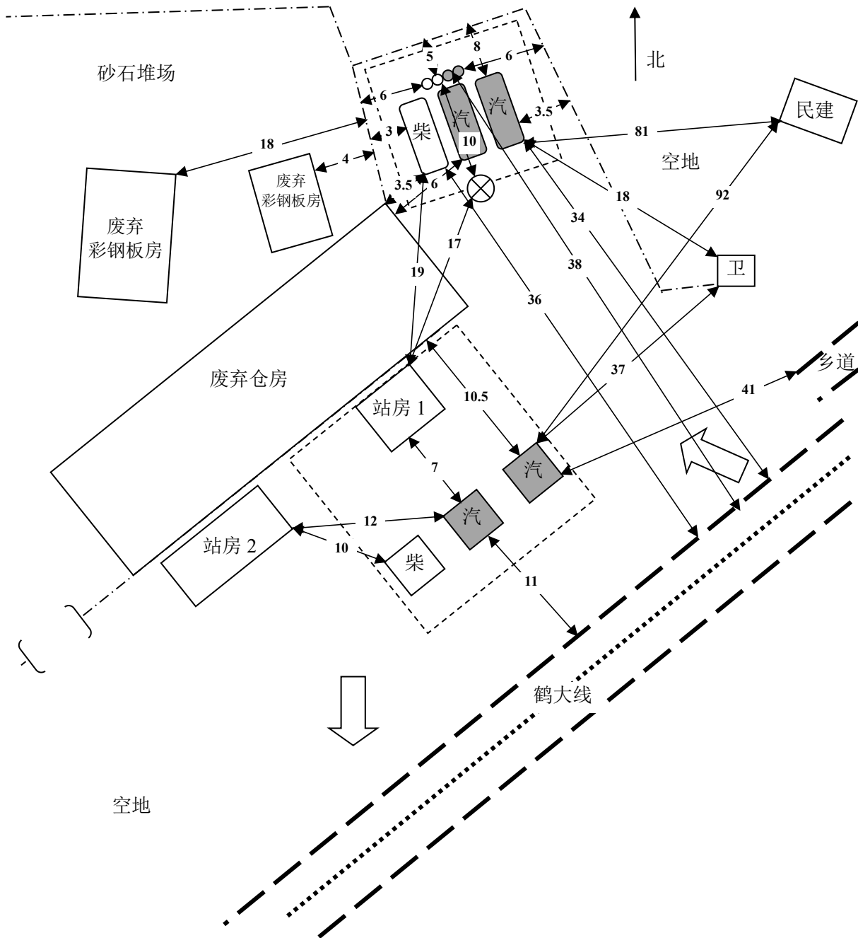
图 2.7.2-1 平面布置图
