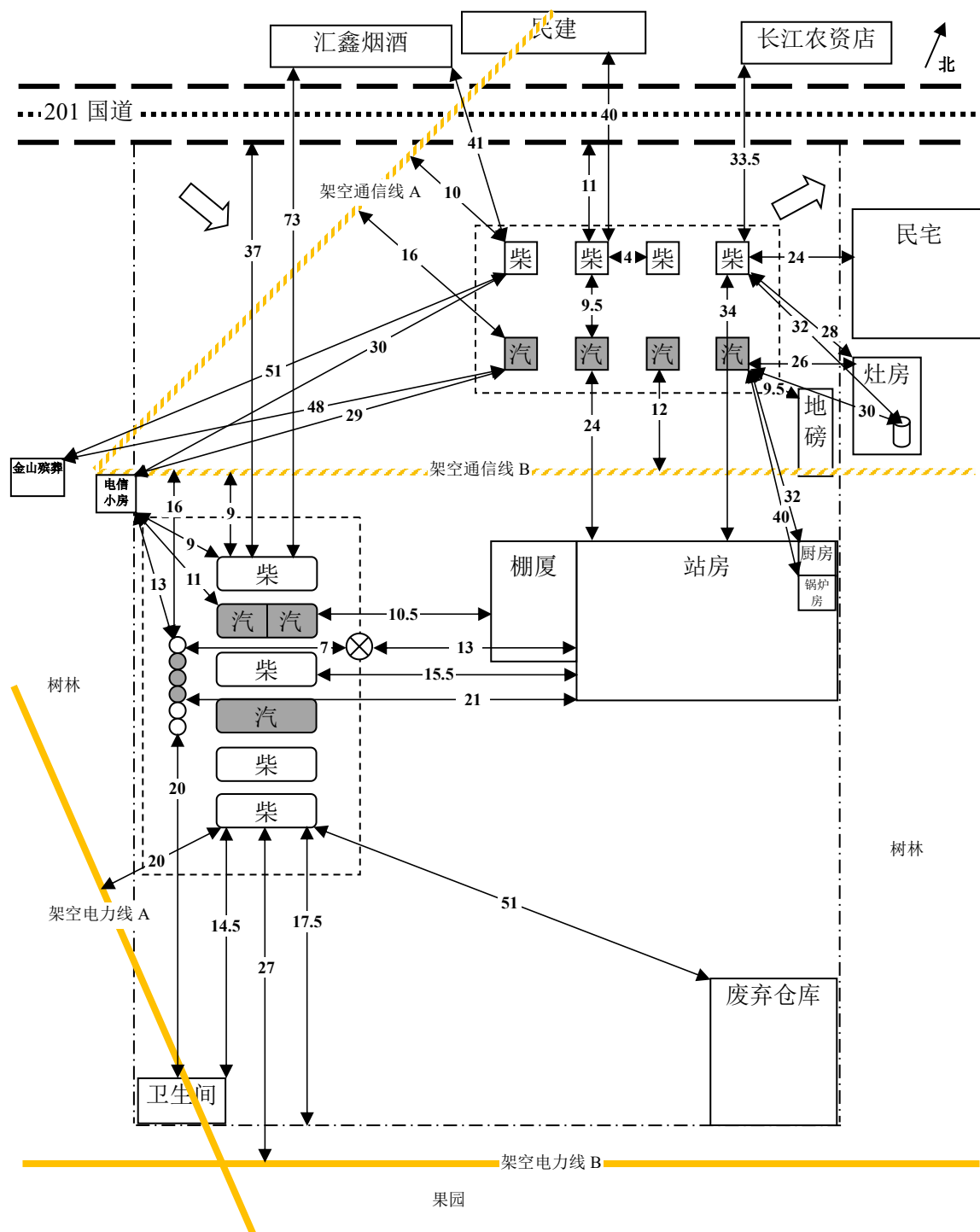
图 2.7.2-1 平面布置图
