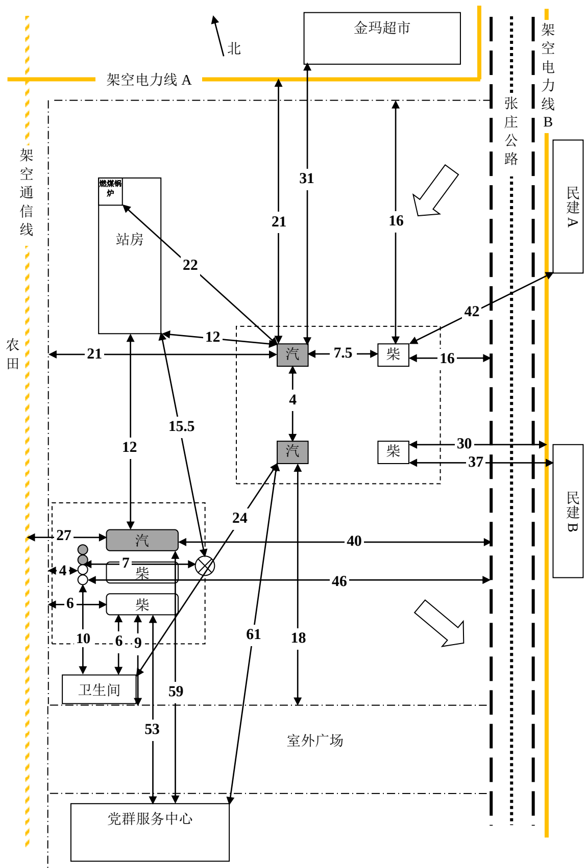
图 2.7.2-1 平面布置图
