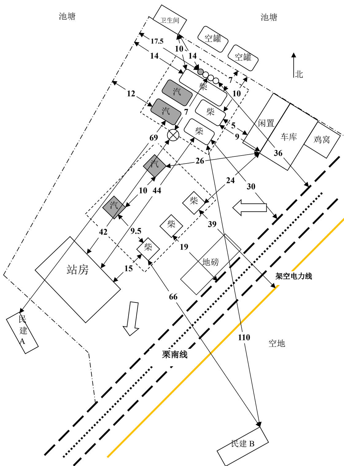
图 2.7.2-1 平面布置图
