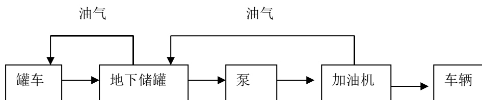
图 2.4.1-1 卸油、加油工艺流程图
