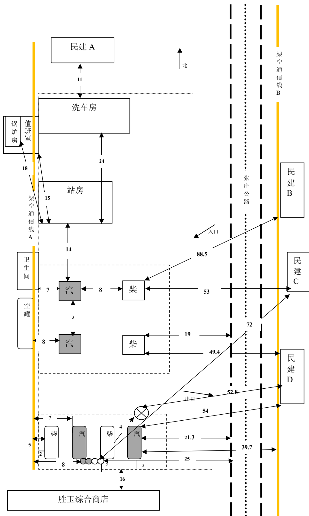
图 2.7.2-1 平面布置图
