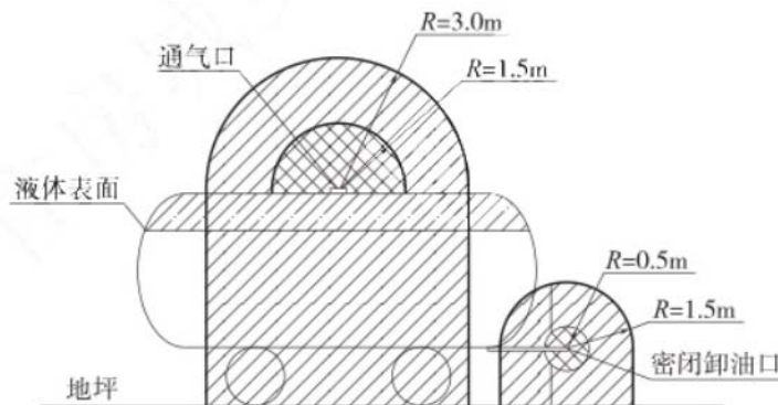
图 C.0.4 汽油油罐车的爆炸危险区域划分
