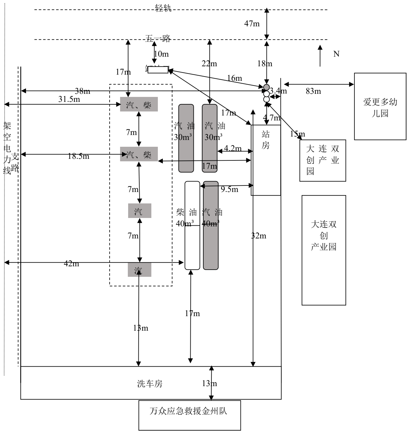
图 2.7.2-1 总平面布置图
