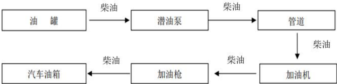
图 2.4.1-4 柴油加油工艺流程图
