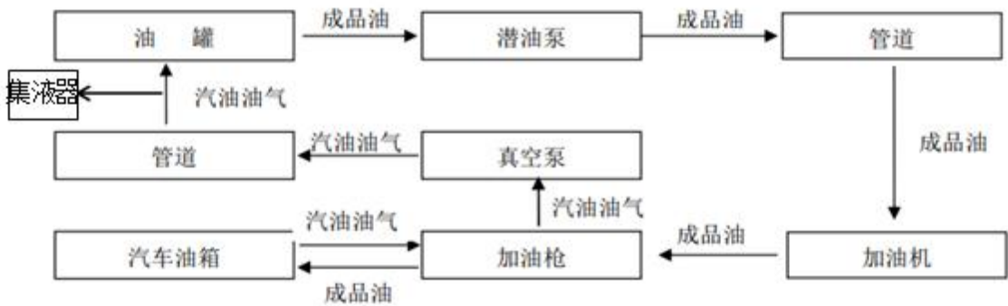
图 2.4.1-3 乙醇汽油加油及油气回收工艺流程图
