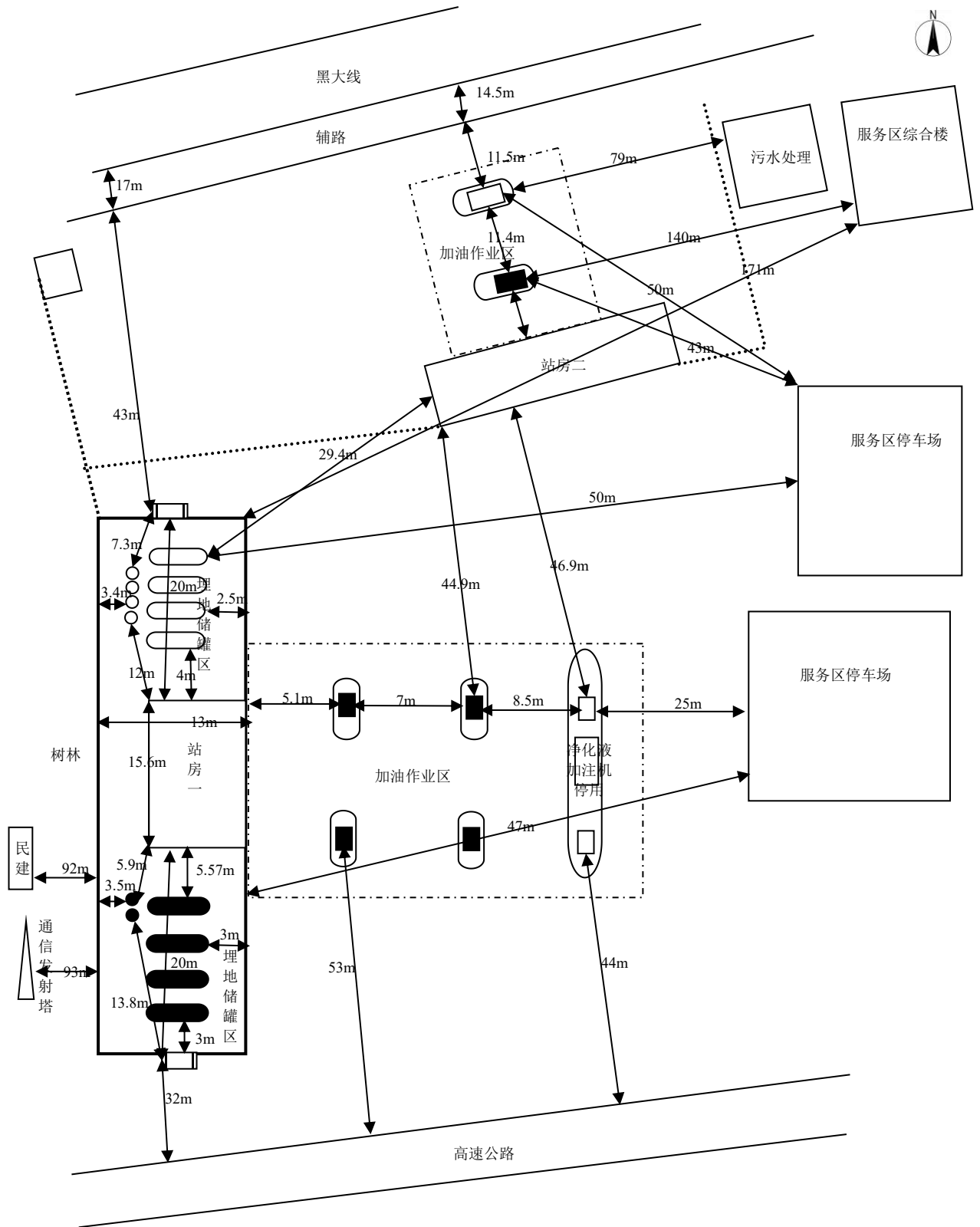
图 2.7.2-1 平面布置图
