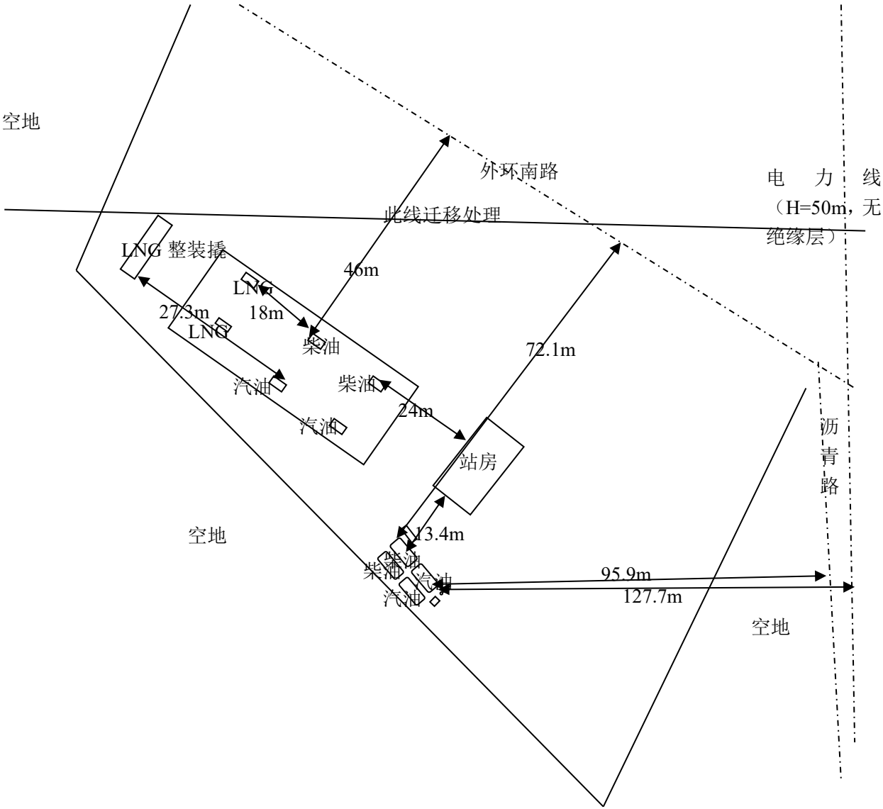
图 2.4.2-1 站区功能布置图
