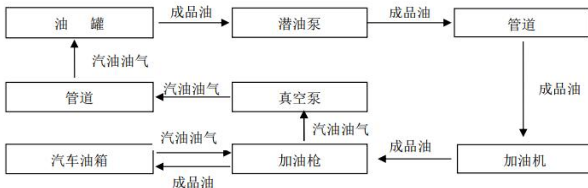
图 2.6.1-3 汽油加油及油气回收工艺流程图
