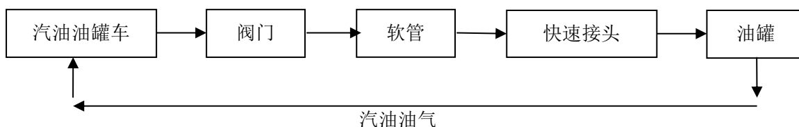
图 2.6.1-1 汽油罐车密闭卸油及汽油油罐卸油油气回收工艺流程图
