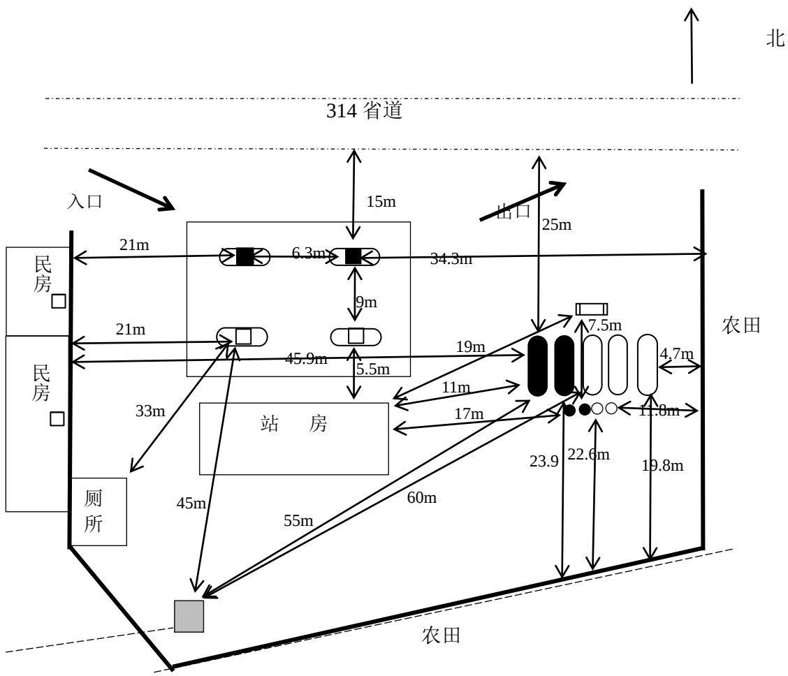
图 2.7.2-1 周边环境及总平面布置图
