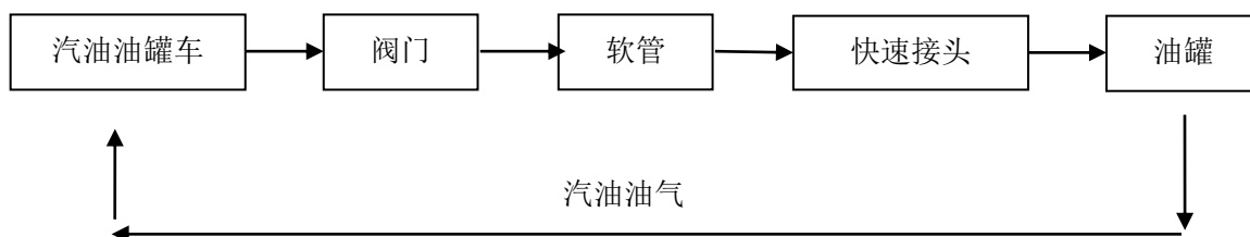
图 2.4.1-1 乙醇汽油罐车密闭卸油及卸油油气回收工艺流程图
