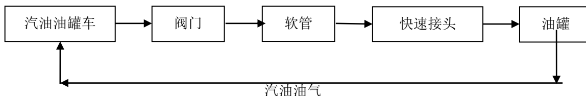
图 2.4.1-1 乙醇汽油罐车密闭卸油及卸油油气回收工艺流程图
