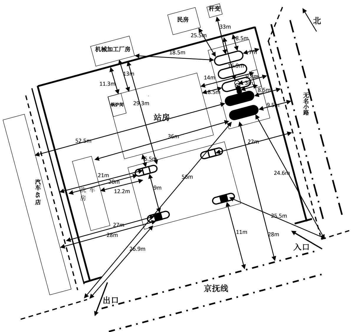
图 2.7.2-1 周边环境及总平面布置图
