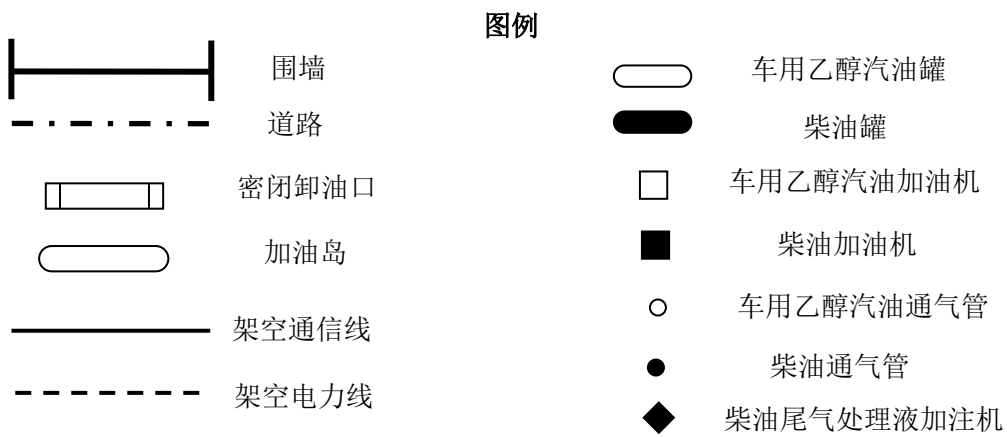
图 2.7.2-1 周边环境及总平面布置图
