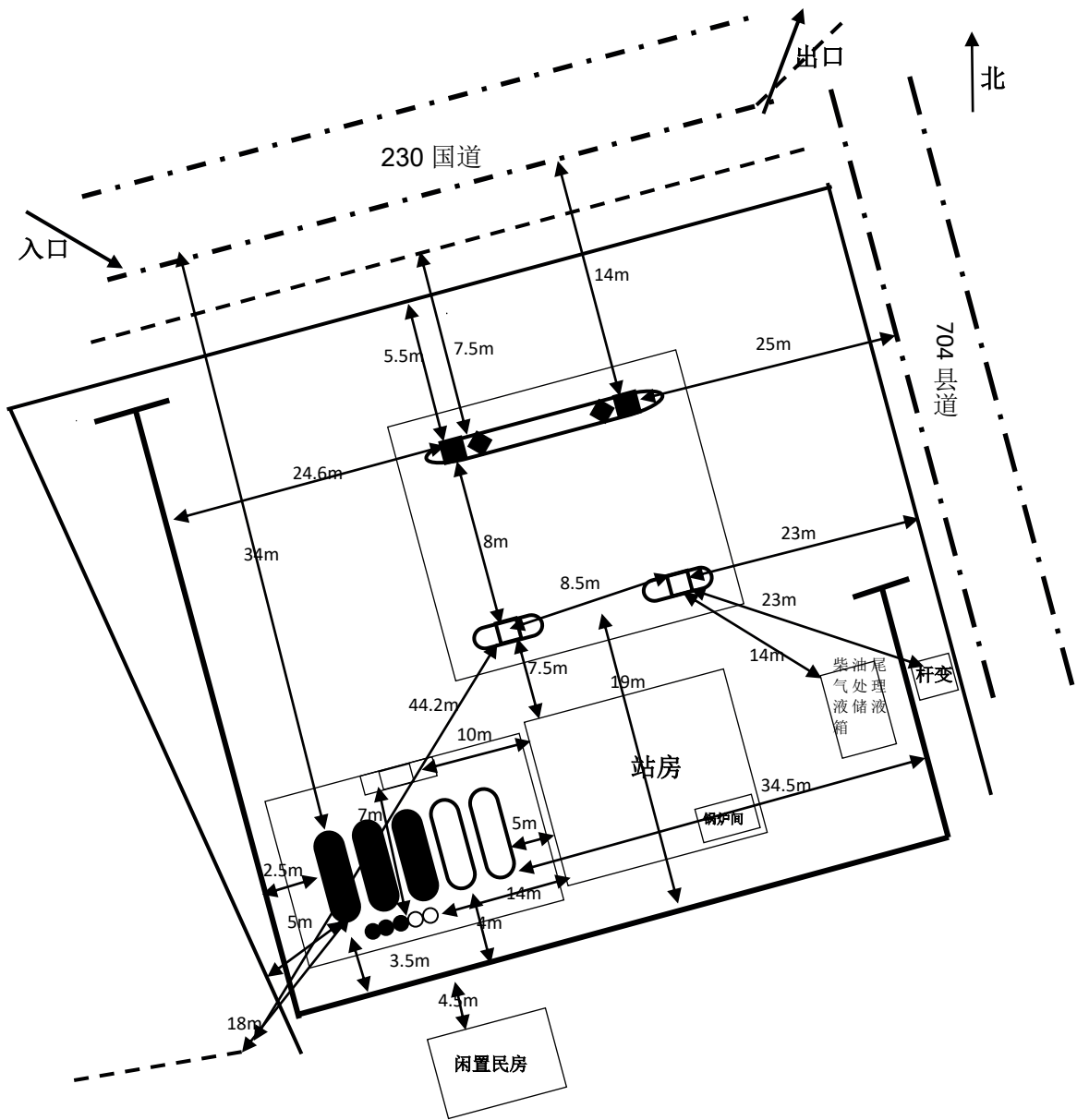
图 2.7.2-1 周边环境及总平面布置图
