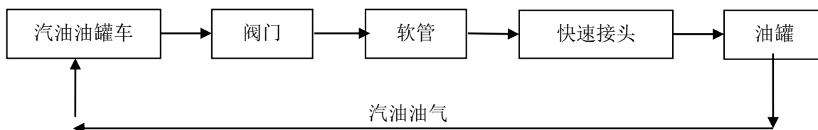
图 2.4.1-1 乙醇汽油罐车密闭卸油及卸油油气回收工艺流程图
