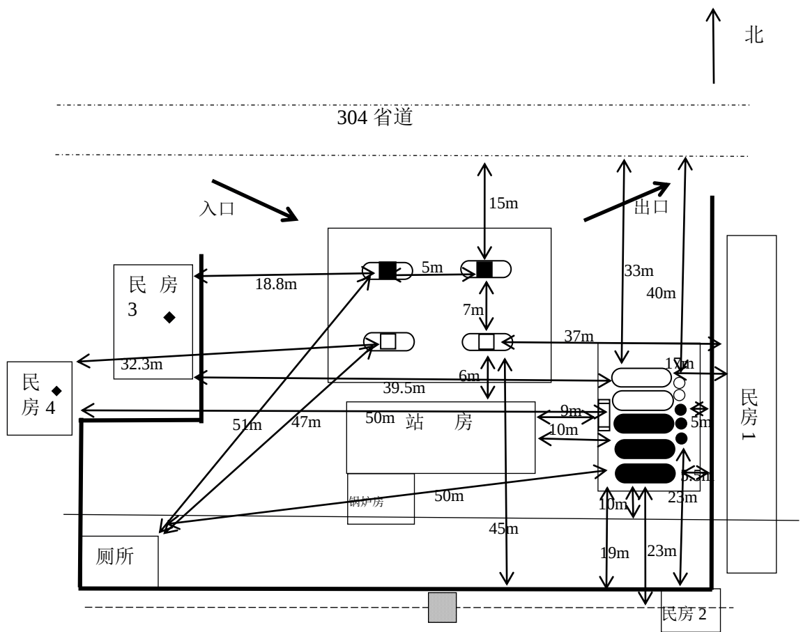
图 2.7.2-1 周边环境及总平面布置图
