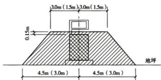
图 C.0.5 汽油加油机的爆炸危险区域划分
