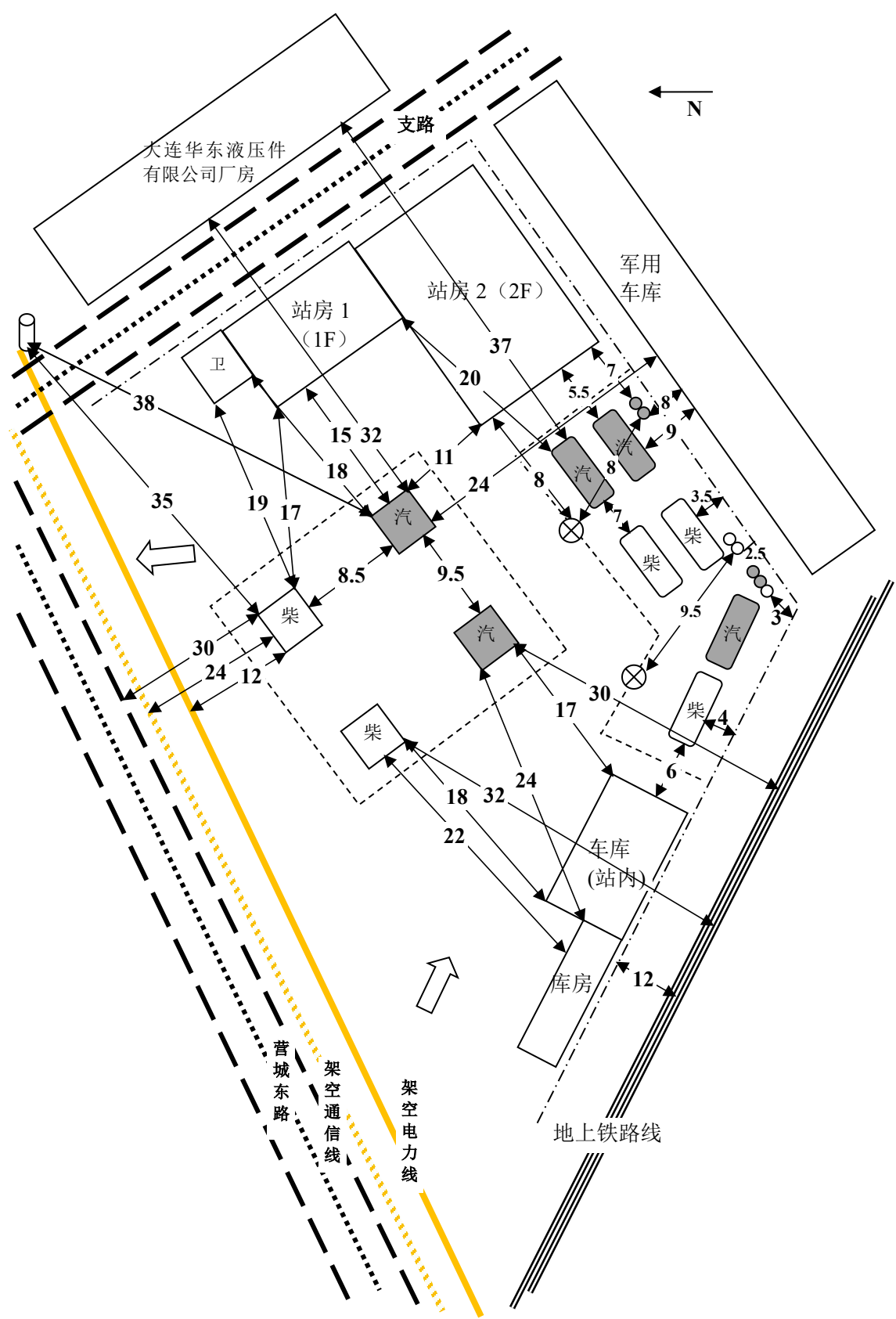
图 2.7.2-1 平面布置图
