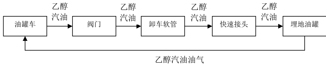
图 2.4.1-1 乙醇汽油罐车密闭卸油及卸油油气回收（一次油气回收）工艺流程图
