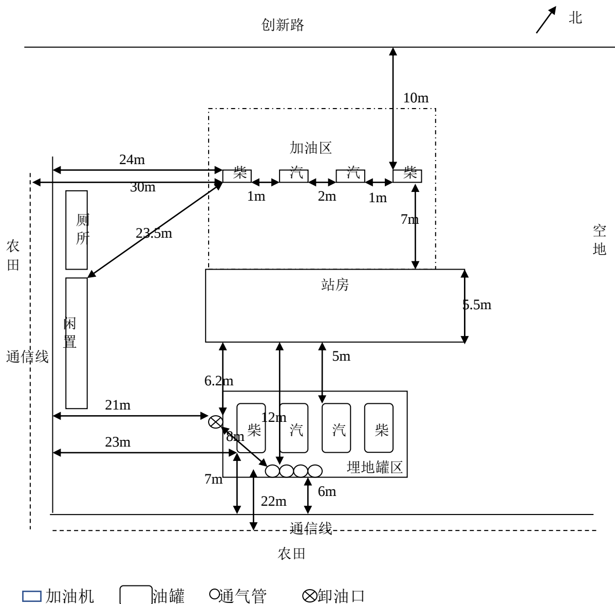
图 2.7.2-1 平面布置图
