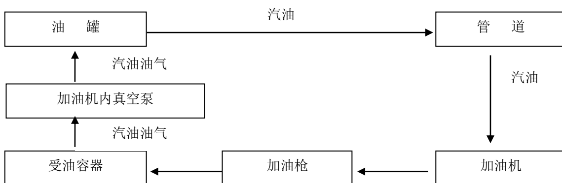
图 2.4.1-3 乙醇汽油加油及油气回收工艺流程图
