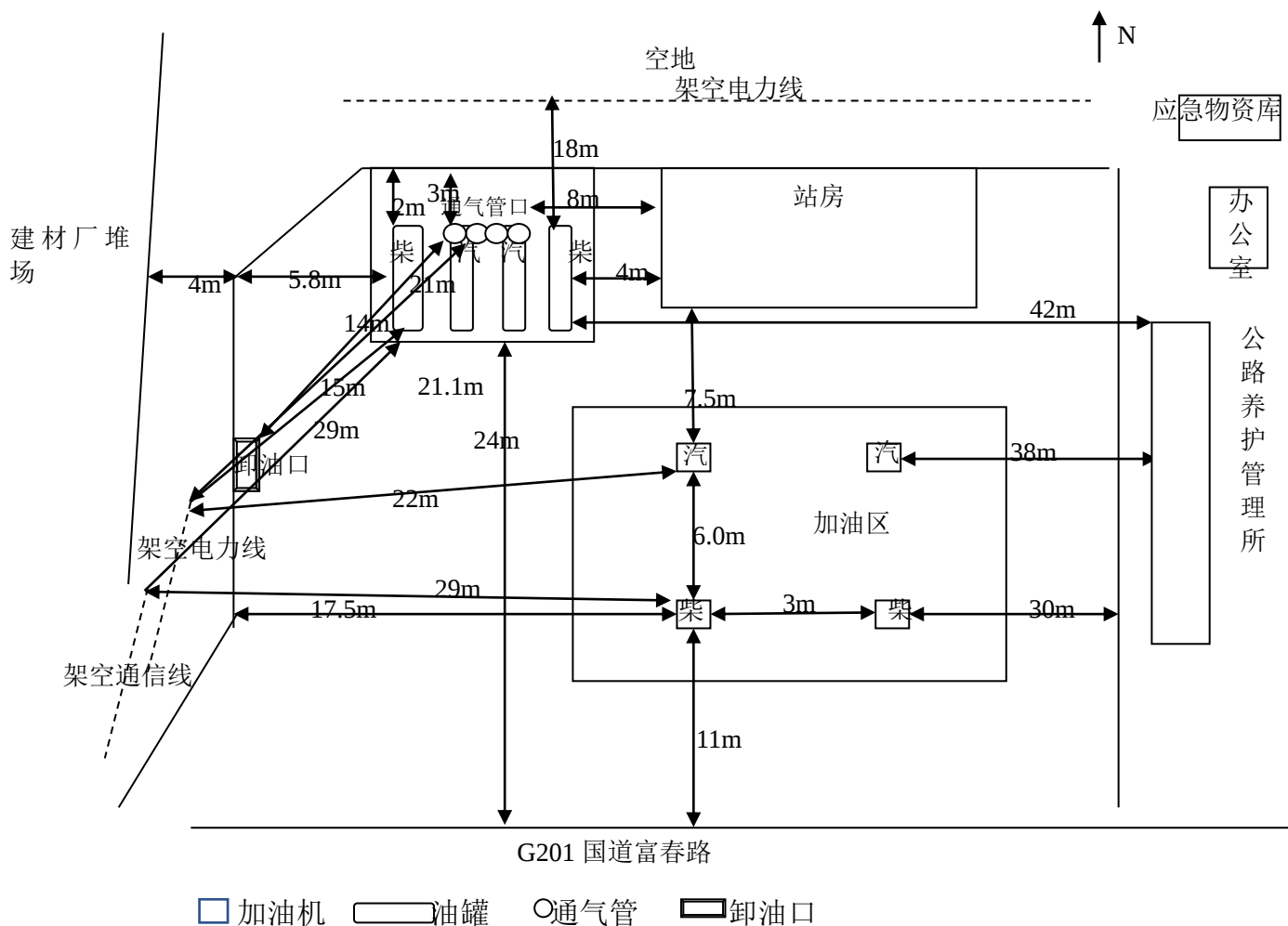
图 2.7.2-1 平面布置图
