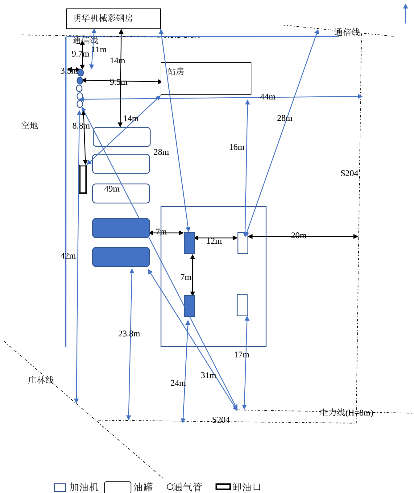
图 2.7.2-1 平面布置图
