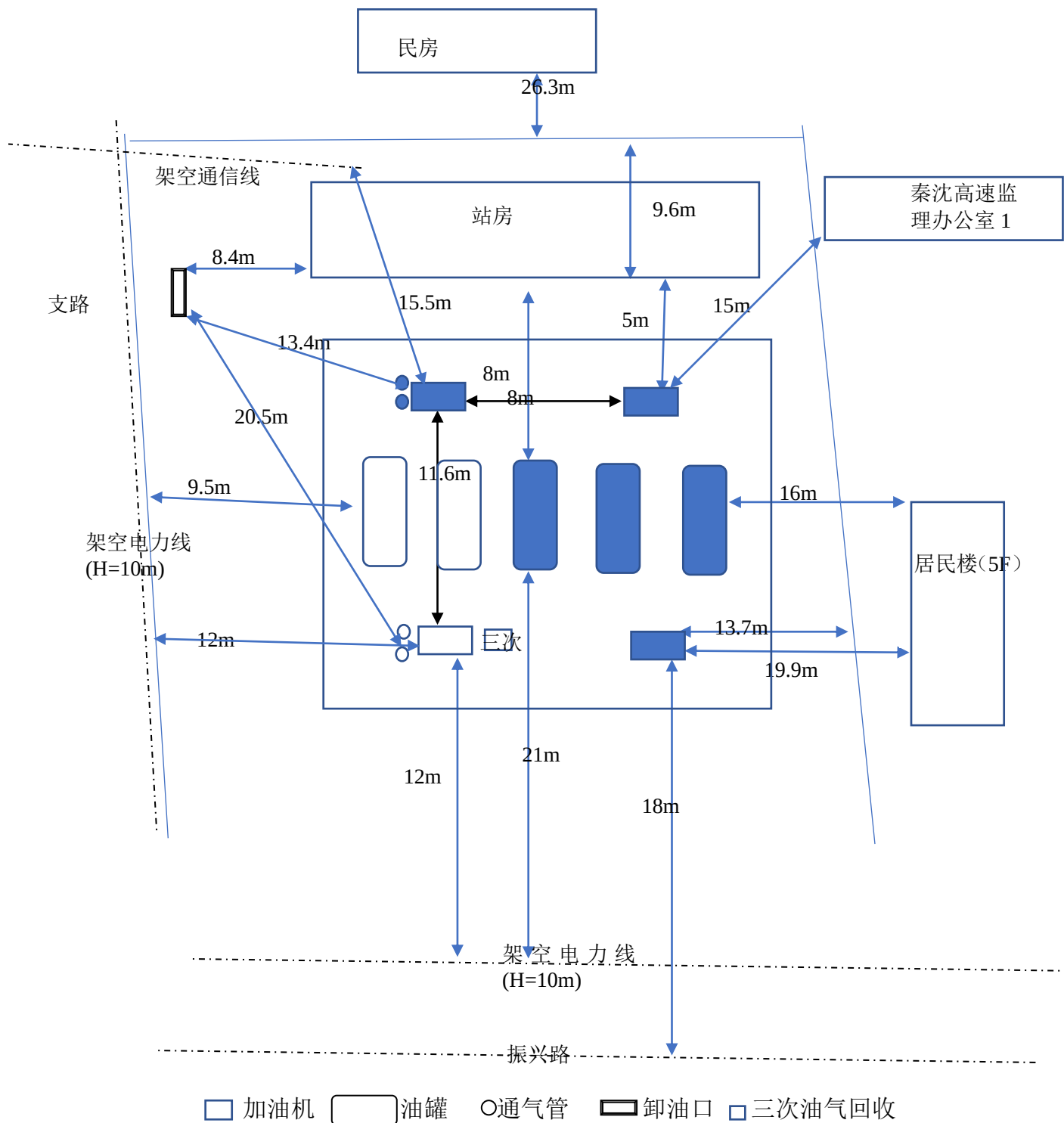
图 2.7.2-1 平面布置图
