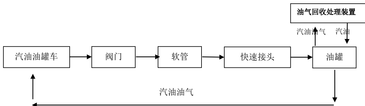
图 2.4.1-1 乙醇汽油罐车密闭卸油及卸油油气回收工艺流程图
