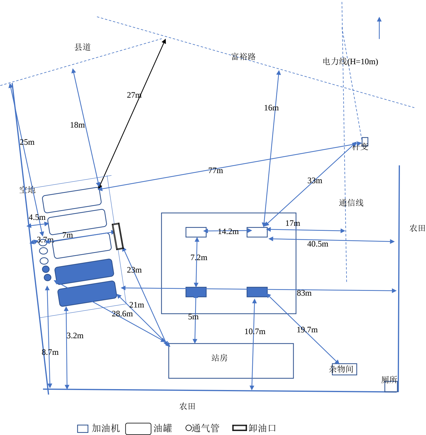
图 2.7.2-1 平面布置图
