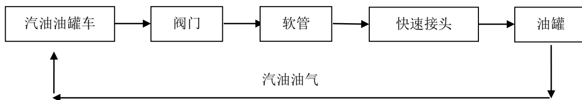
2.4.1-1 乙醇汽油罐车密闭卸油及卸油油气回收工艺流程图
