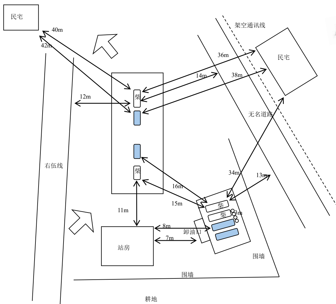
图 2.7.2-1 平面布置图
