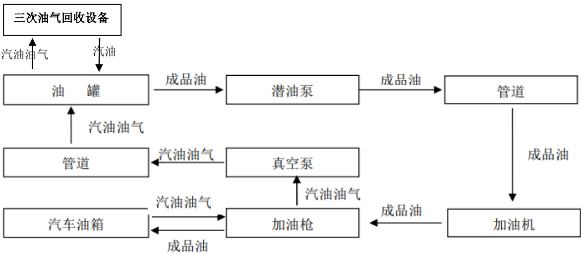
图 2.4.1-2 乙醇汽油加油及油气回收工艺流程图
