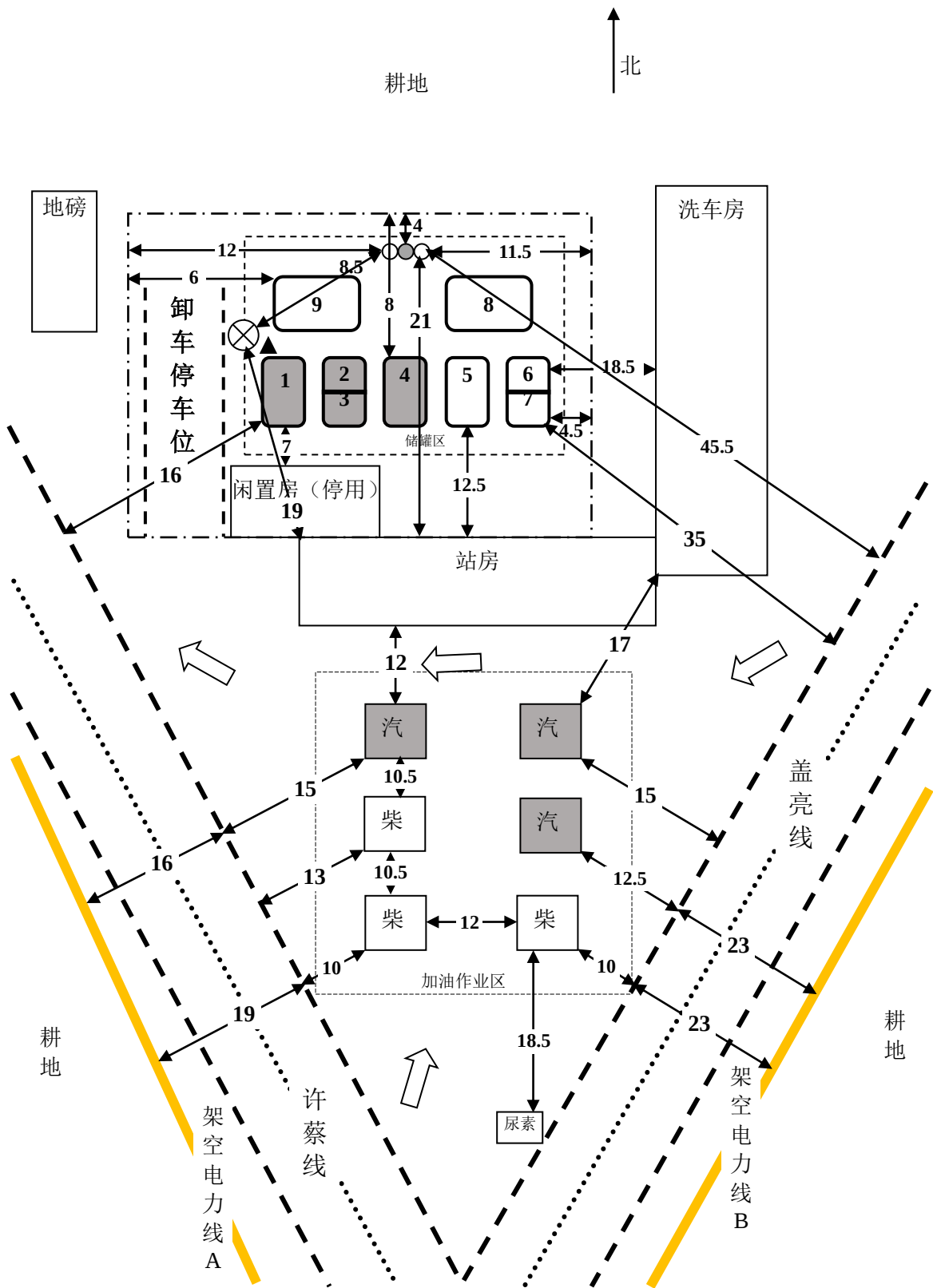
图 2.7.2-1 平面布置图
