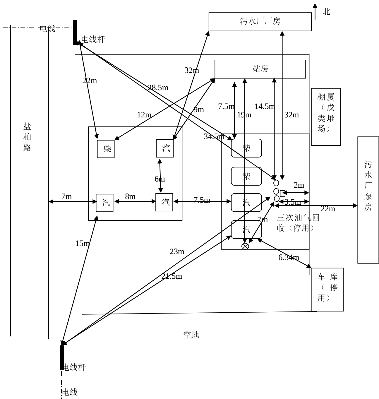
图 2.7.2-1 平面布置图
