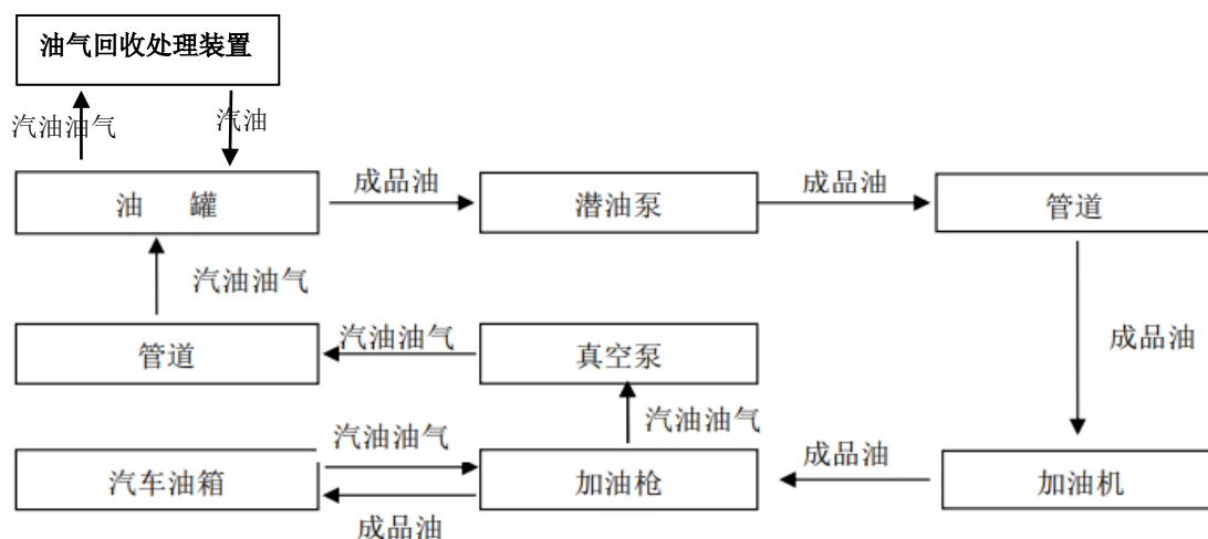
图 2.4.1-2 乙醇汽油加油及油气回收工艺流程图
