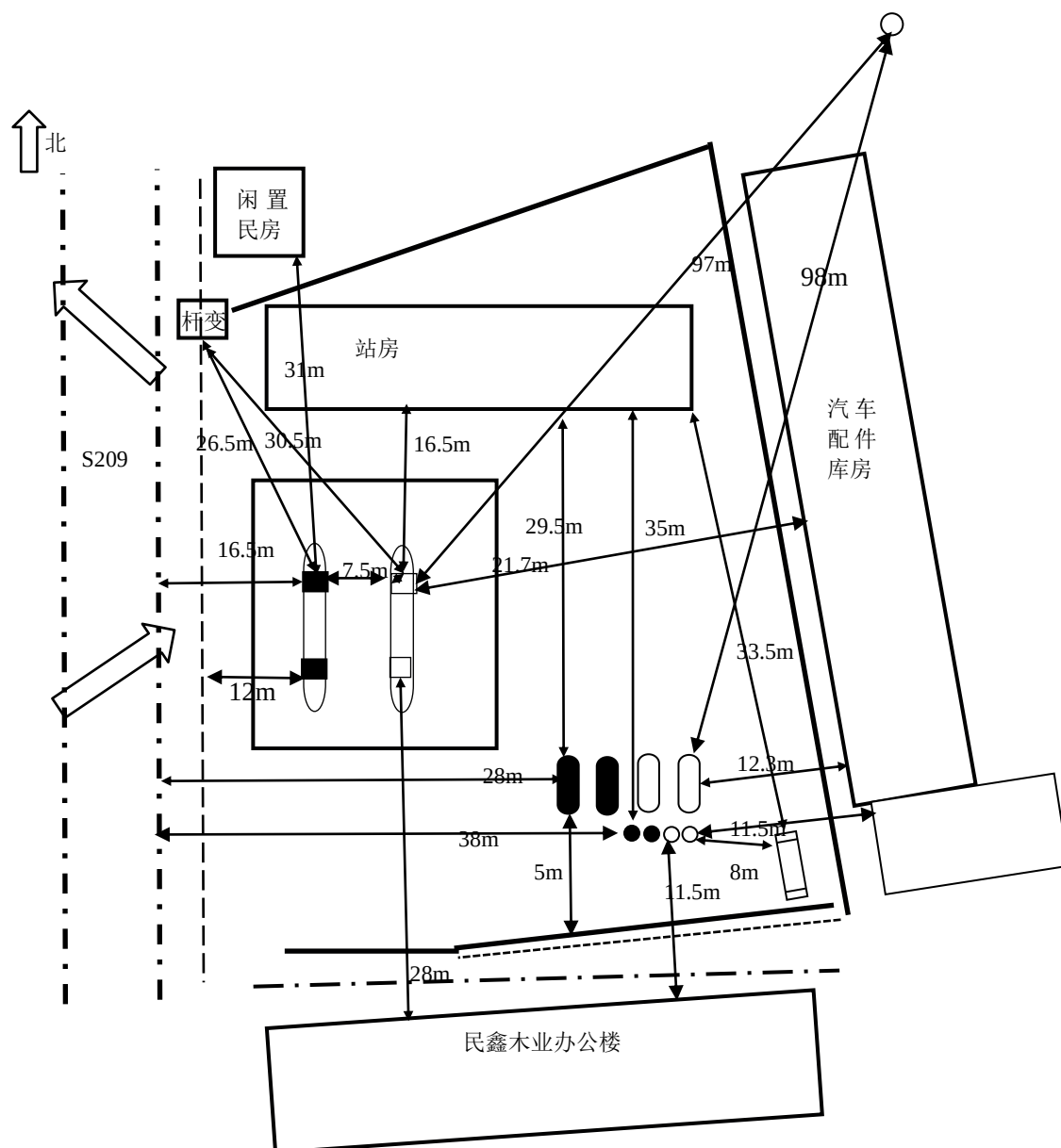
图 2.7.2-1 平面布置图
