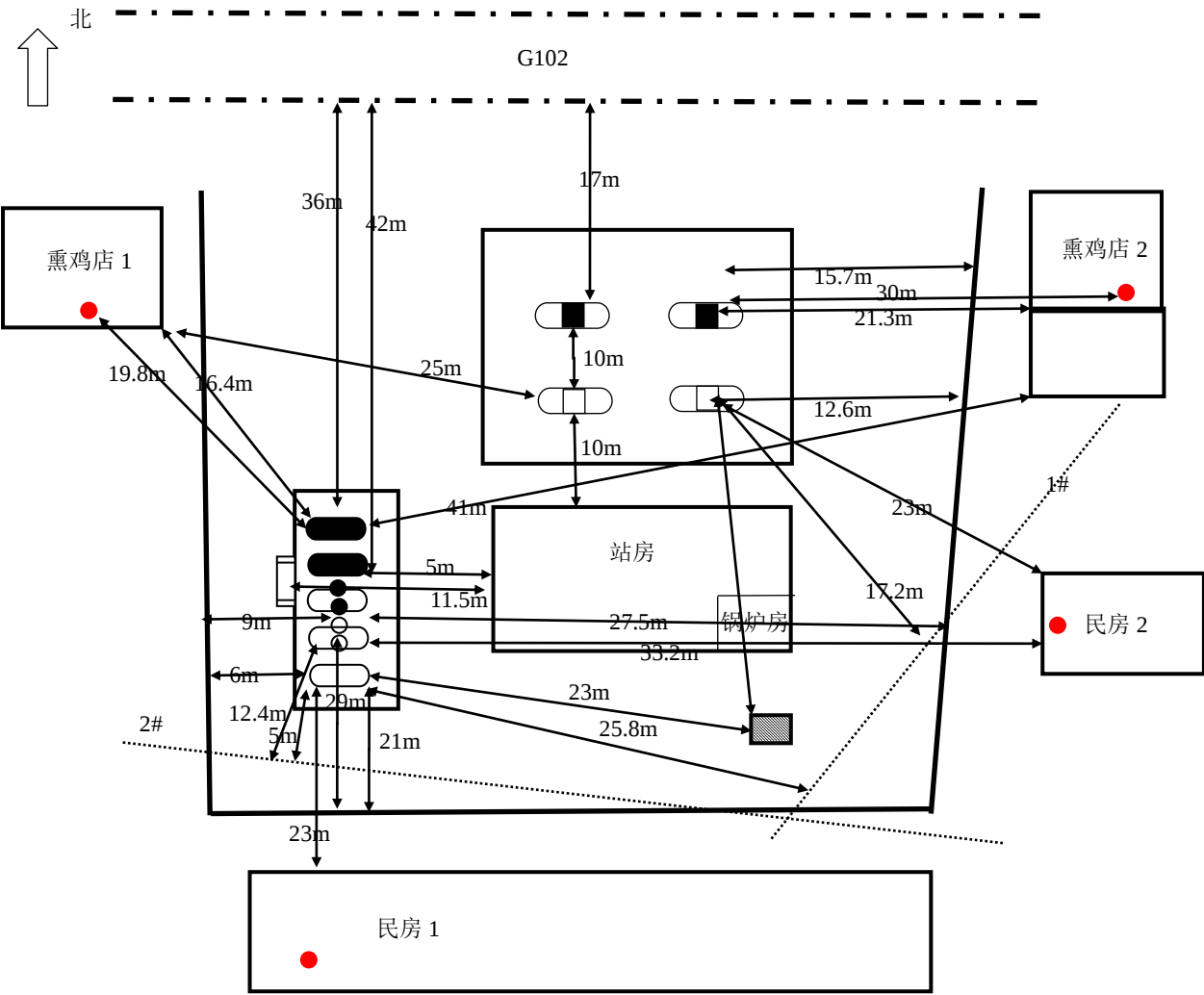
图 2.7.2-1 周边环境及总平面布置图
