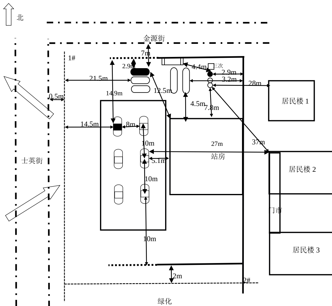
图 2.7.2-1 平面布置图
