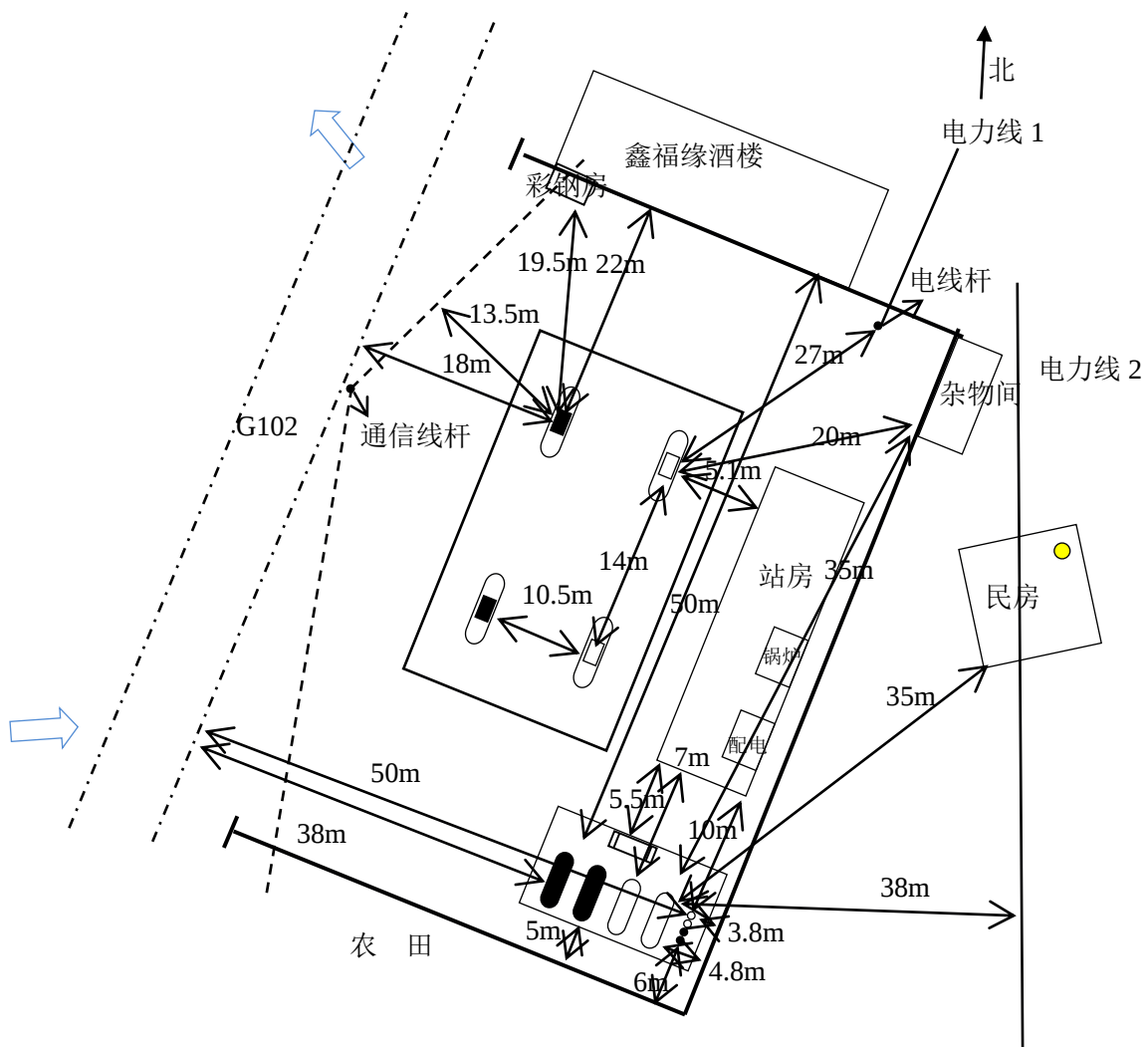
图 2.7.2-1 平面布置图
