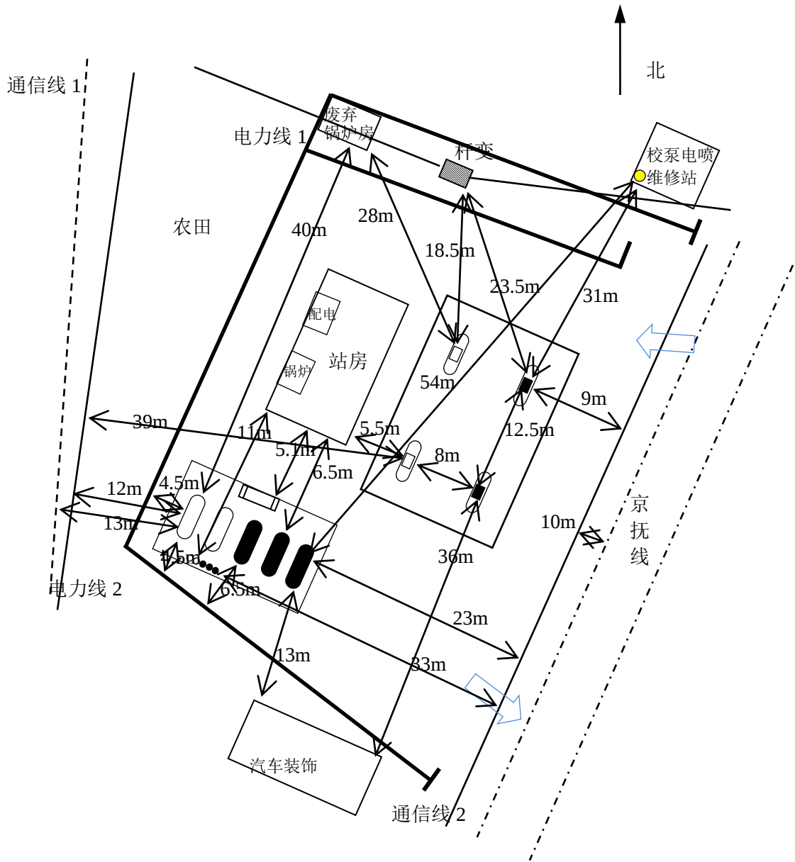
图 2.7.2-1 平面布置图
