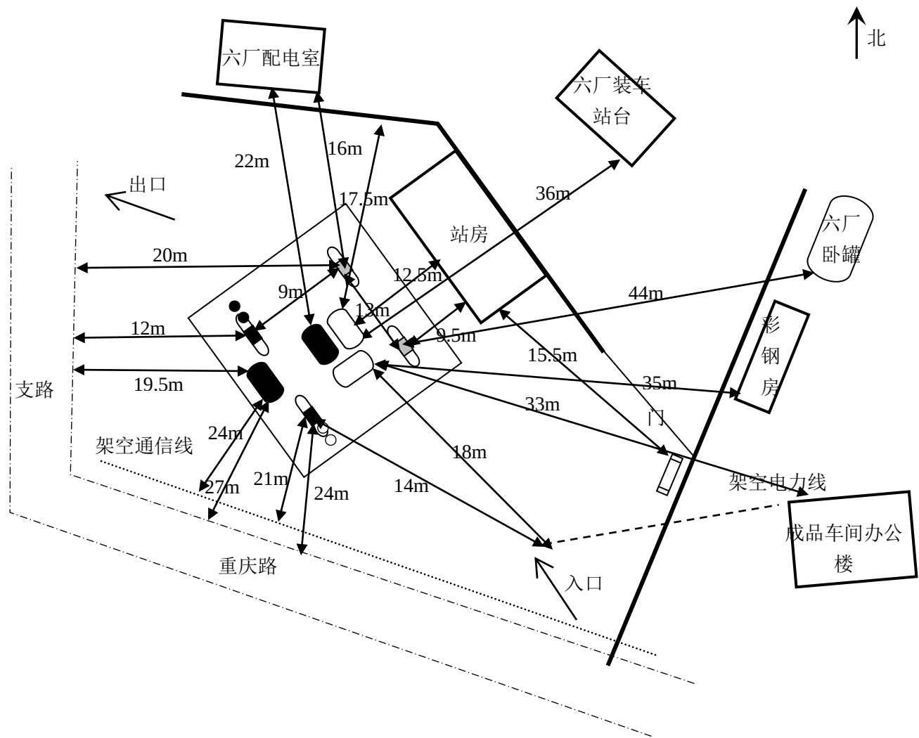
图 2.7.2-1 平面布置图 图 例
