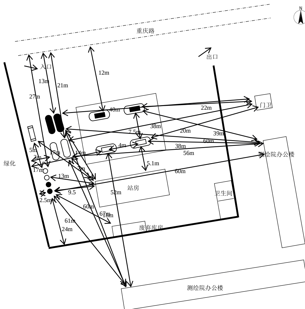
图 2.7.2-1 平面布置图
