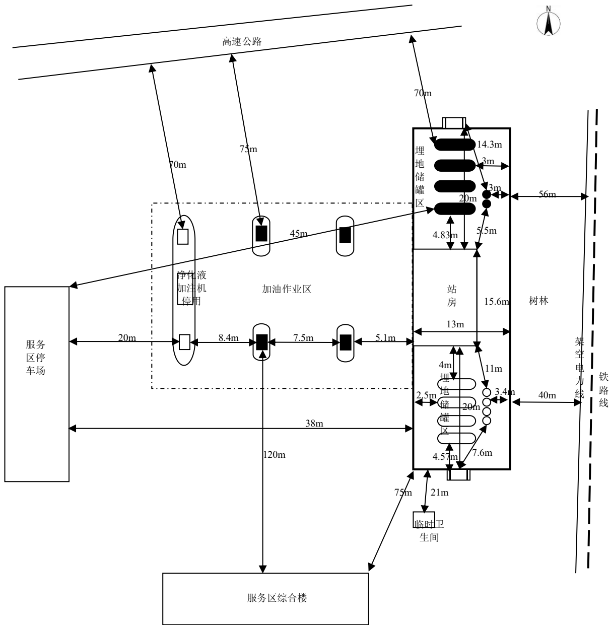
图 2.7.2-1 平面布置图
