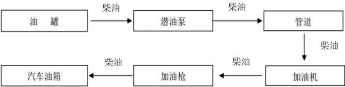
图 2.4.1-4 柴油加油工艺流程图
