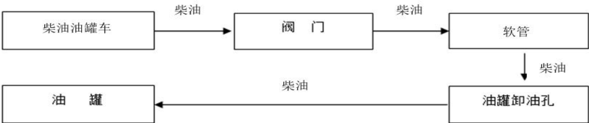
图 2.4.1-2 柴油罐车密闭卸油工艺流程图
