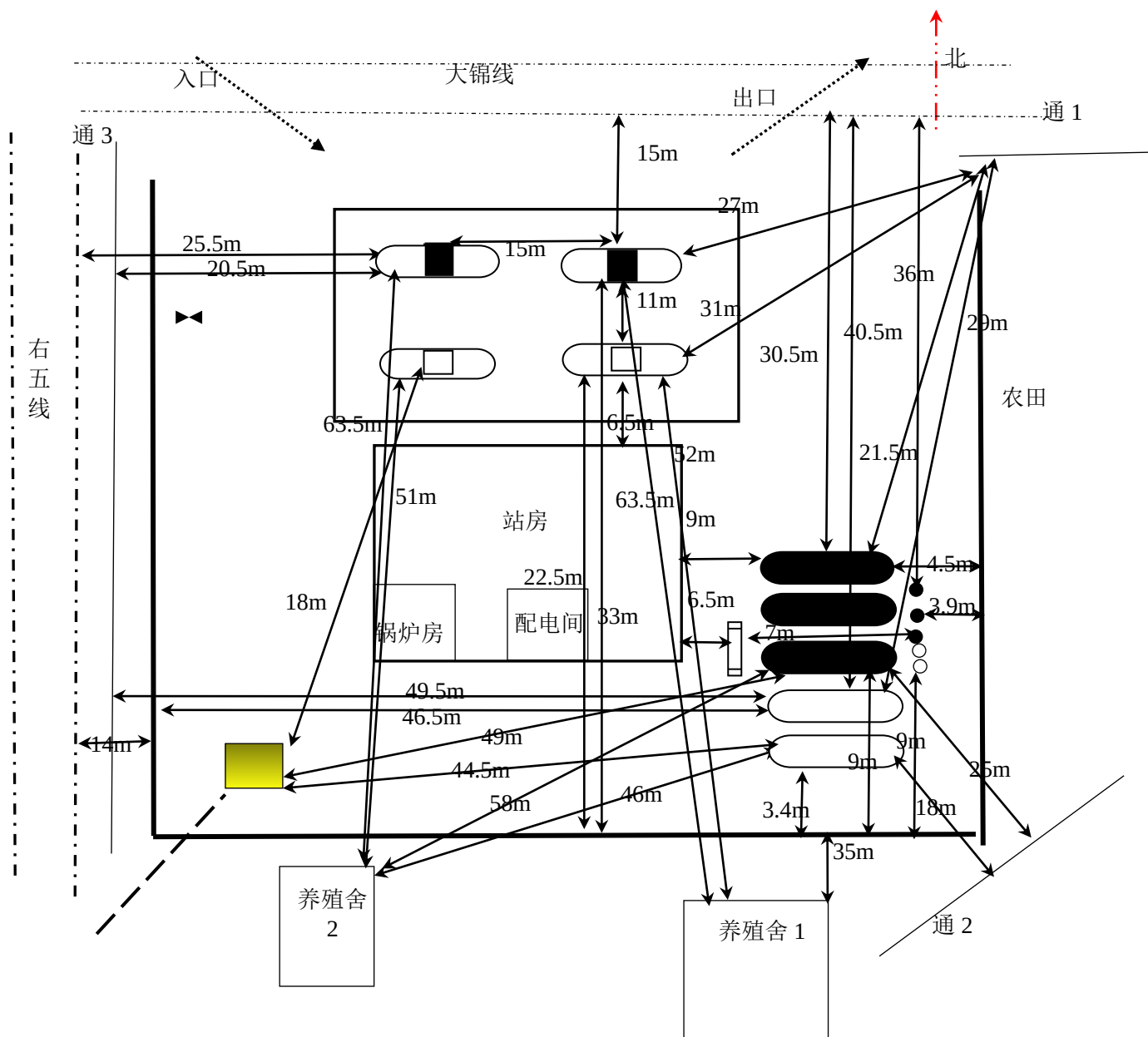
图 2.7.2-1 周边环境及总平面布置情况
