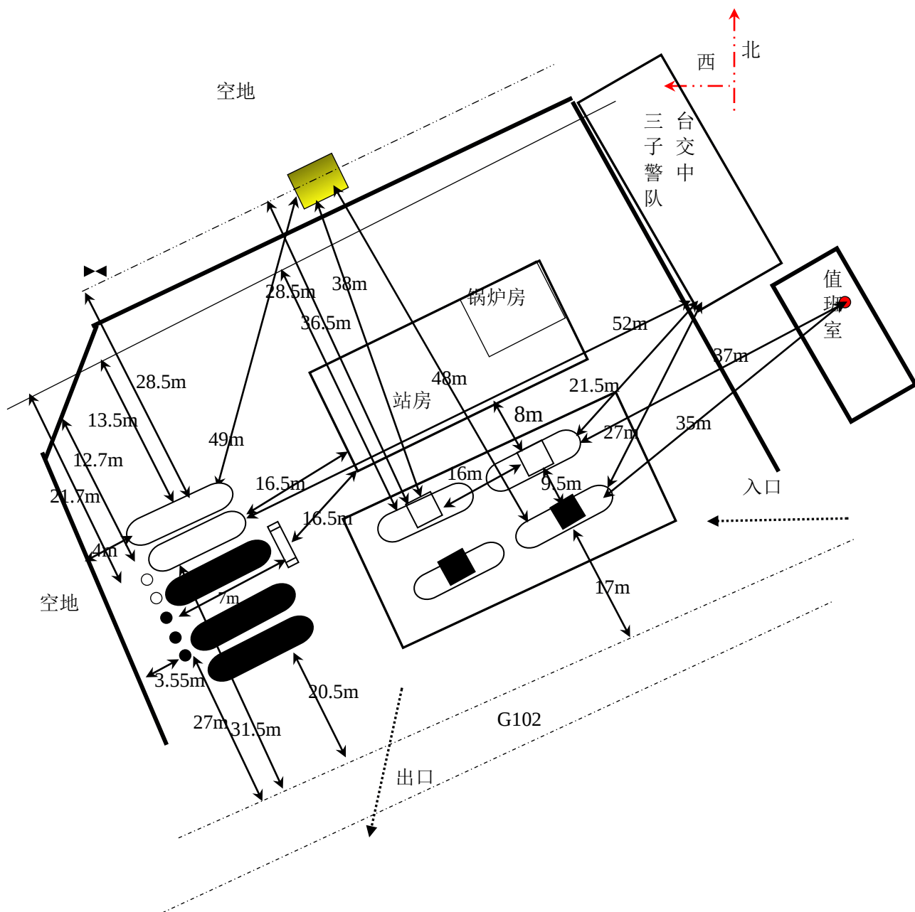
图 2.7.2-1 周边环境及总平面布置情况
