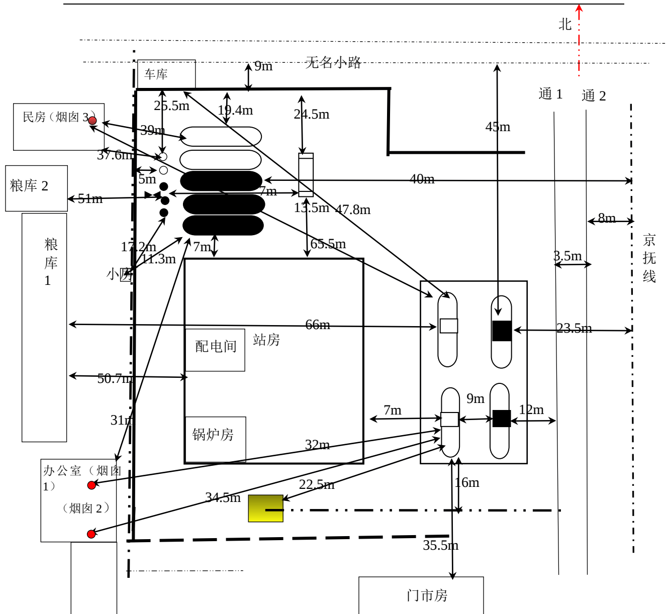
图 2-1 周边环境及总平面布置情况
