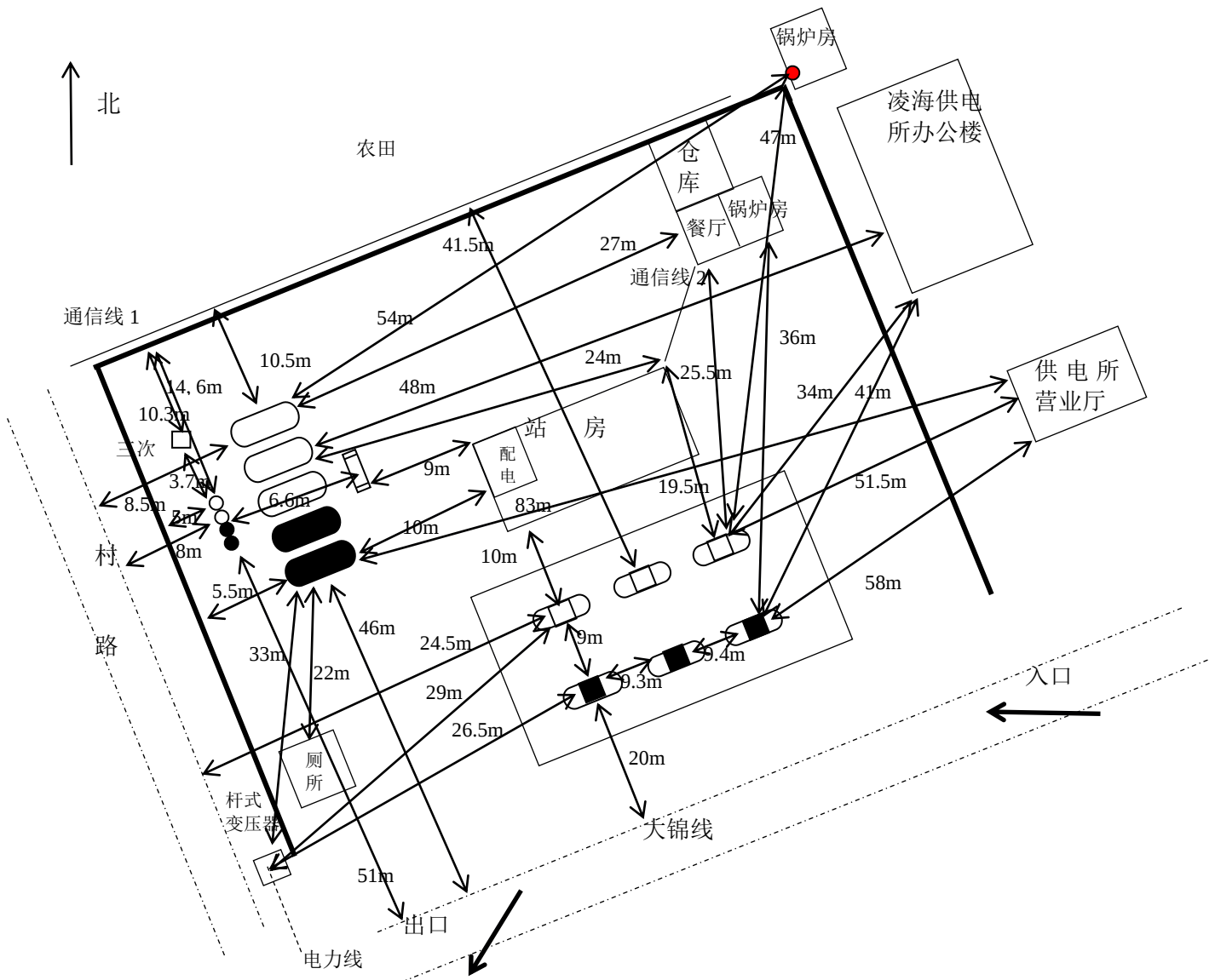
图 2.7.2-1 周边环境及总平面布置图
