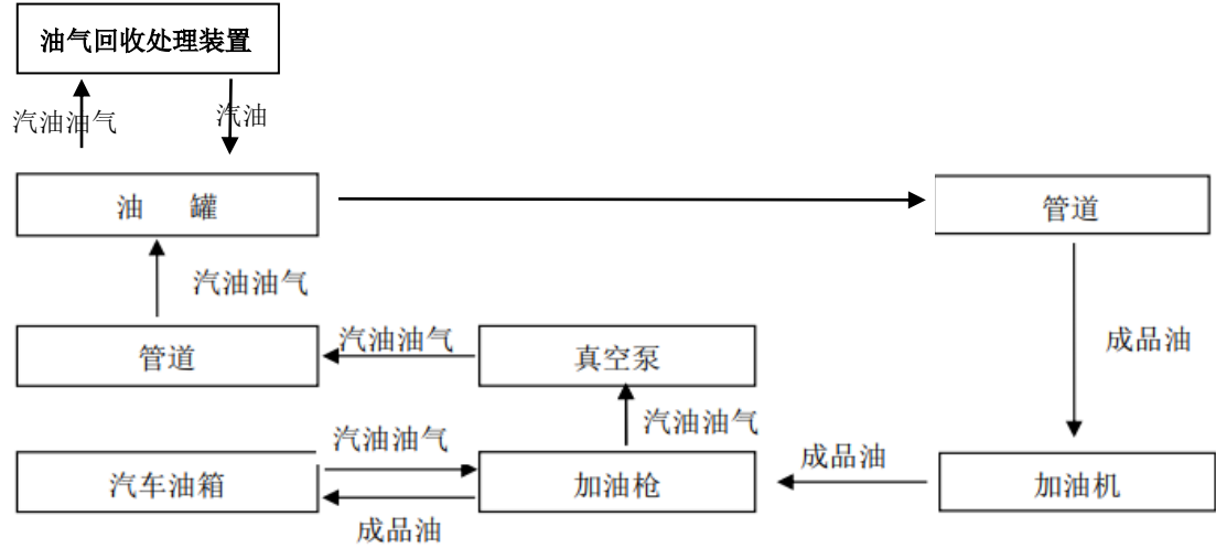
图 2.4.1-3 乙醇汽油加油及油气回收工艺流程图
