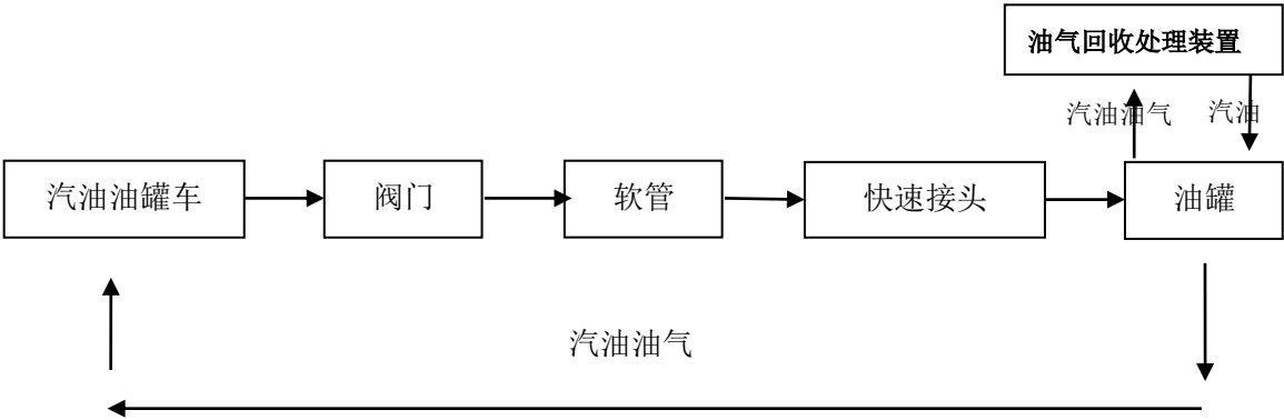
图 2.4.1-1 乙醇汽油罐车密闭卸油及卸油油气回收工艺流程图
