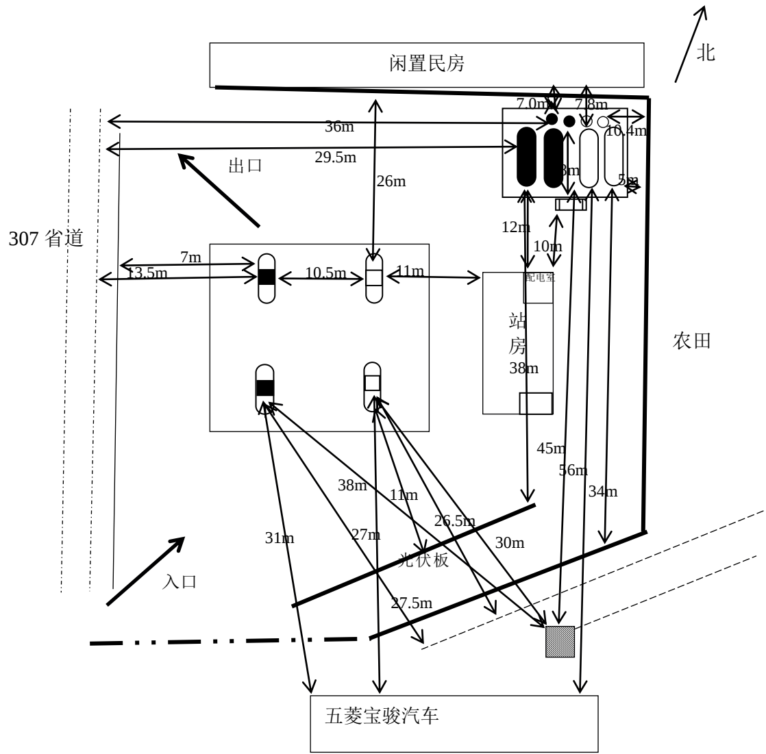
图 2.7.2-1 周边环境和总平面布置图
