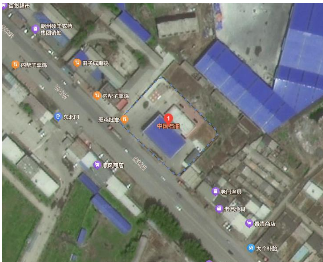
图 2.7.1-1 卫星图
