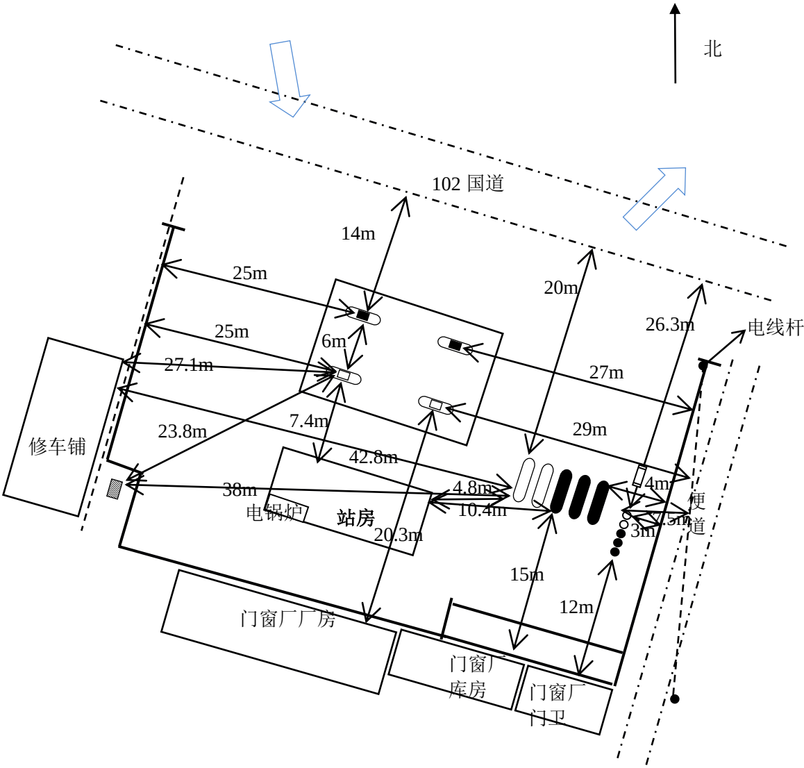
图 2.7.2-1 周边环境及总平面布置图
