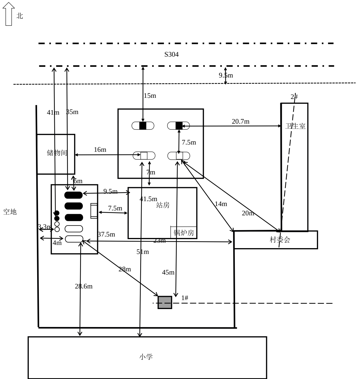
图 2.7.2-1 周边环境及总平面布置图 图例
