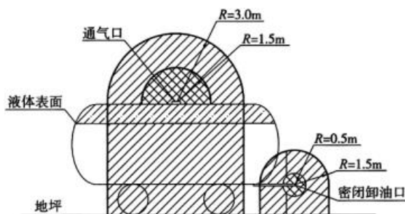
图 C.0.4 汽油油罐车的爆炸危险区域划分
