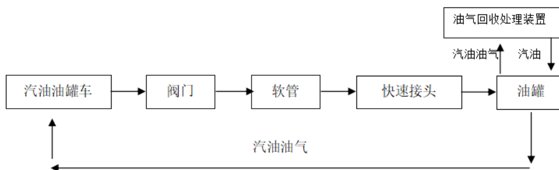
图 2.4.1-1 乙醇汽油罐车密闭卸油及卸油油气回收工艺流程图
