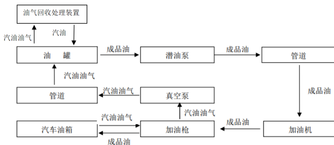
图 2.4.1-3 乙醇汽油加油及油气回收工艺流程图
