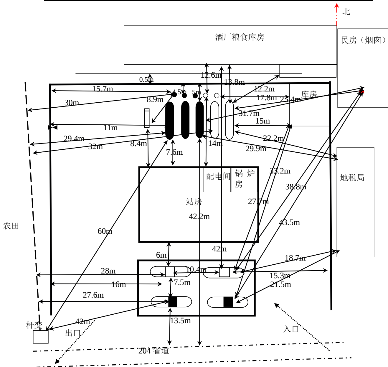
图 2.7.2-1 周边环境及总平面布置情况
