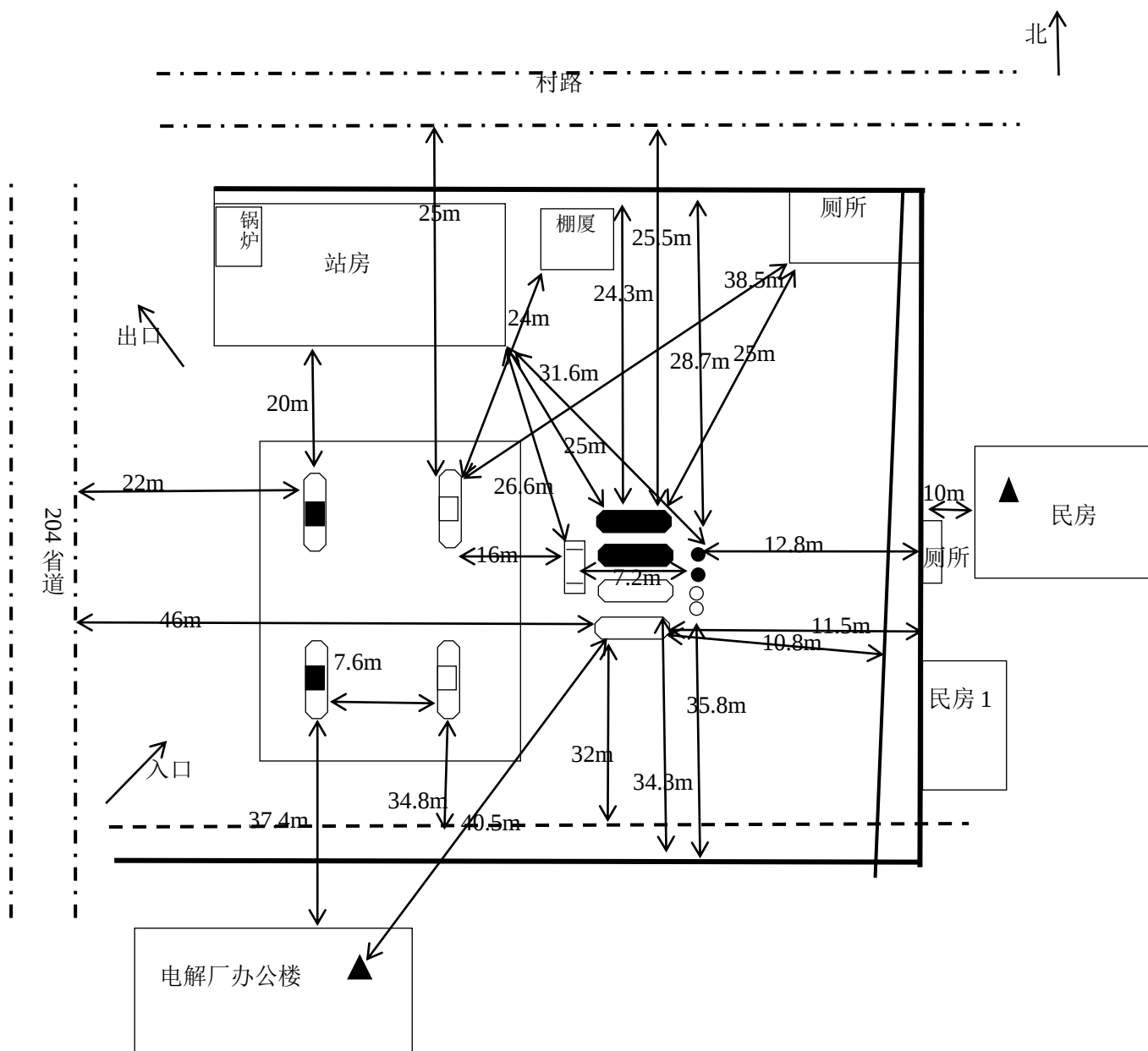
图 2.7.2-1 周边环境及总平面布置图
